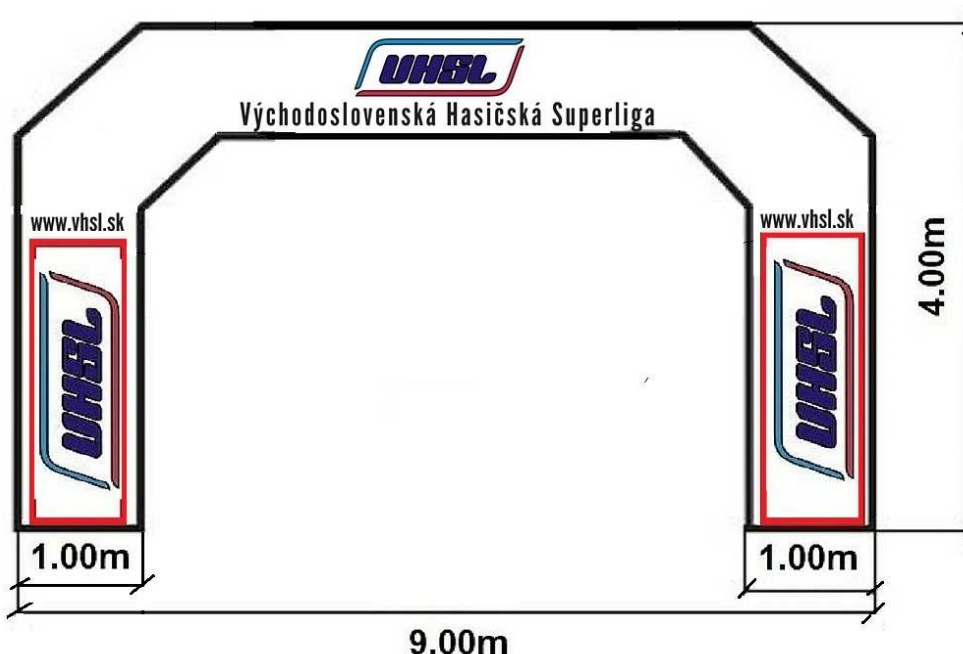
Obrázok 1 Navrhnutý vizuál nafukovacieho oblúku VHSL s rozmermi
